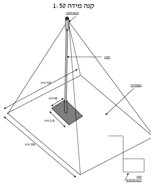
12.2.20 תרשימי רפסודה – ייצוב התורן
