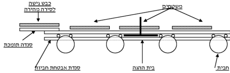
12.2.19 תרשימי רפסודה – מבט צד אחורי
